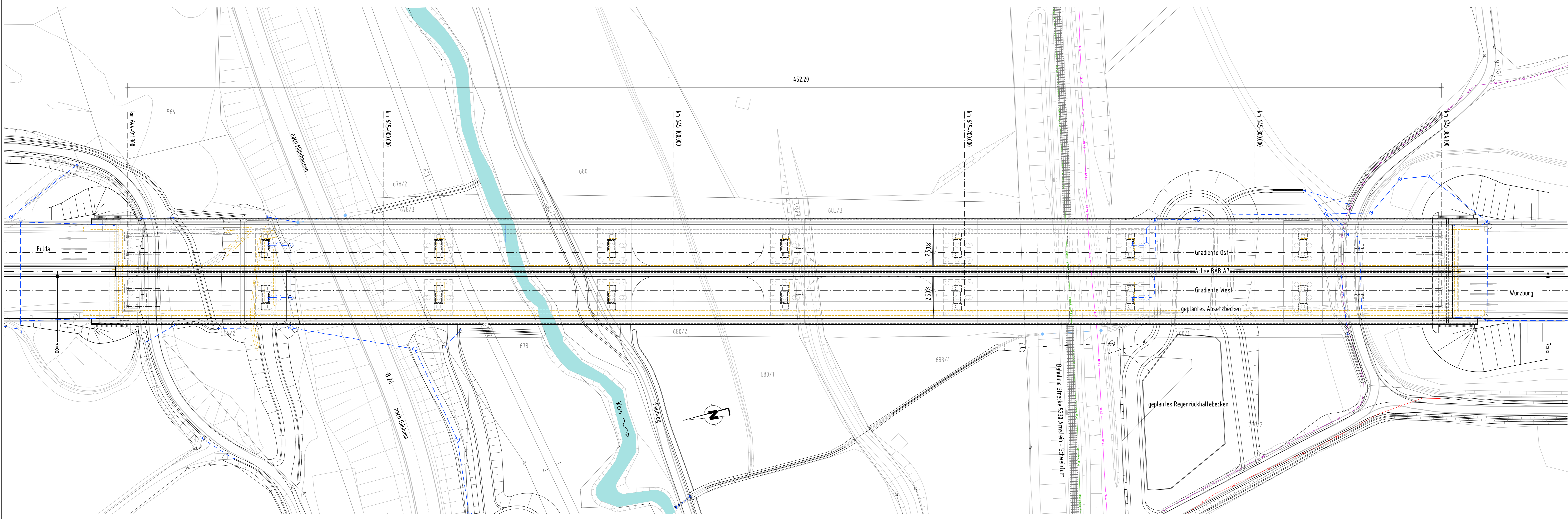
Draufsicht M 1:500
