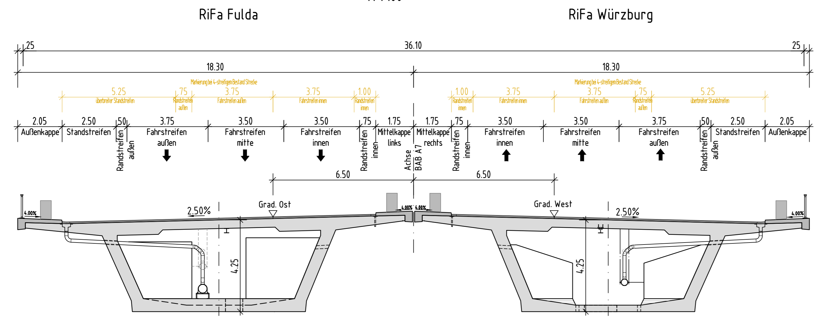
Regelquerschnitt (RQ 36 B) M 1:100
